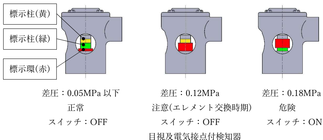
スイッチ(電気接点付検知器)の定格
